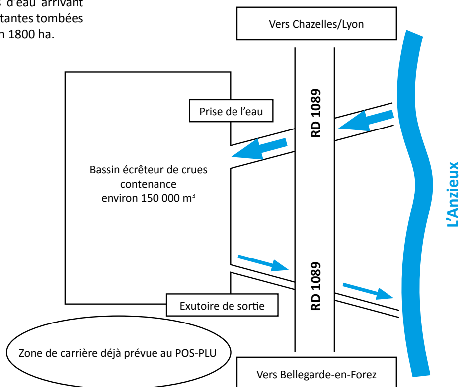
Schéma de principe de l'ouvrage dynamique, écrêteur de crues
